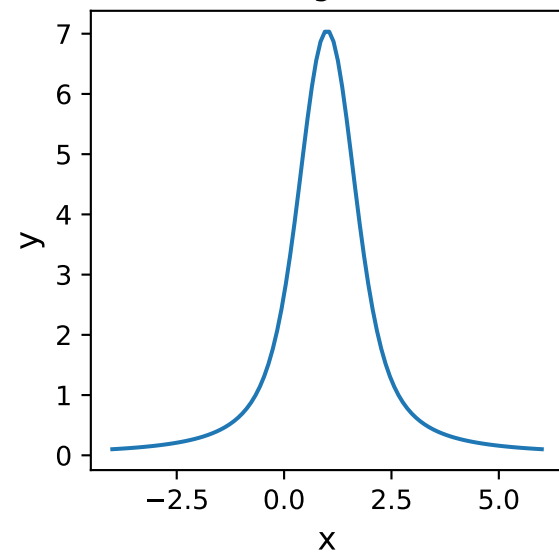
Voigt1D
