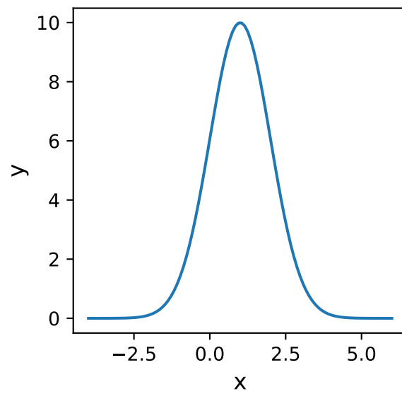
Gaussian1D
